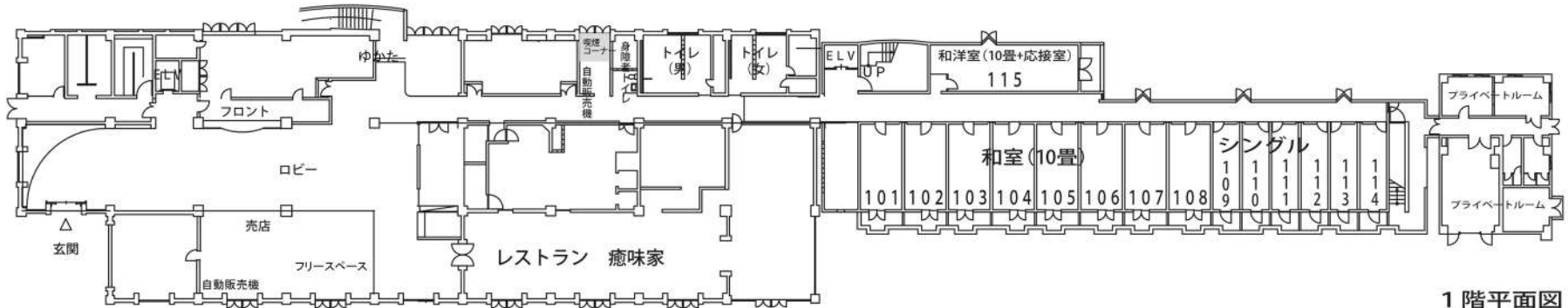
1階平面図
